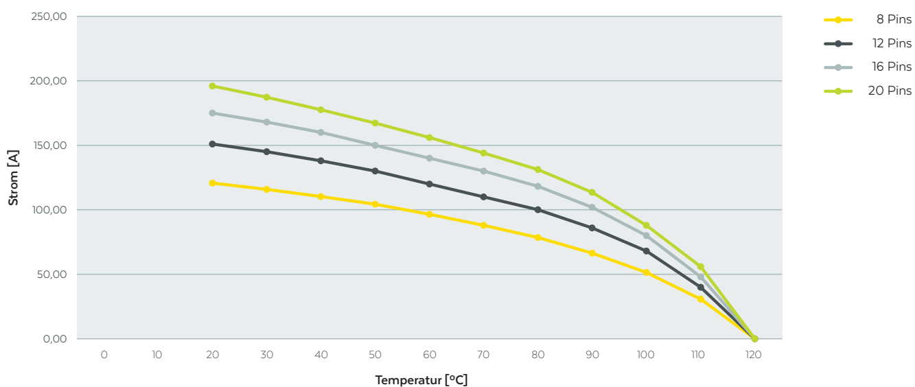
Derating Messung für Power Line massiv rundum
