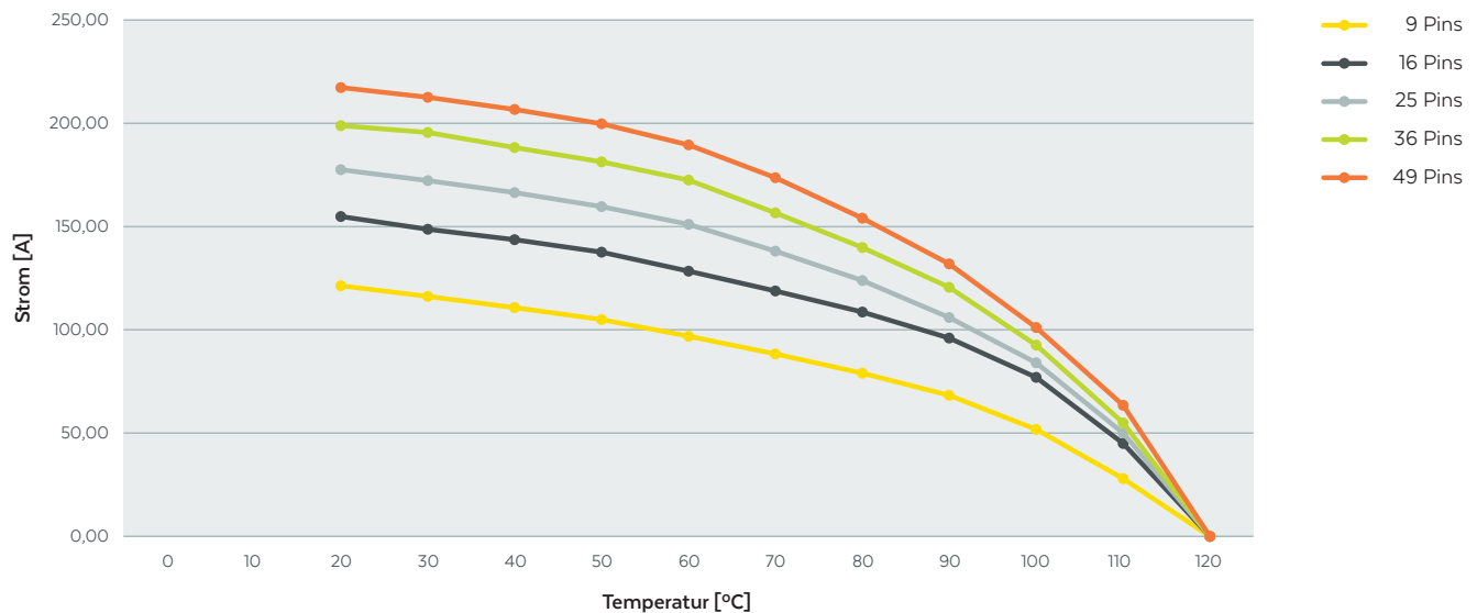
Derating Messung für Power Line massiv vollflächig
