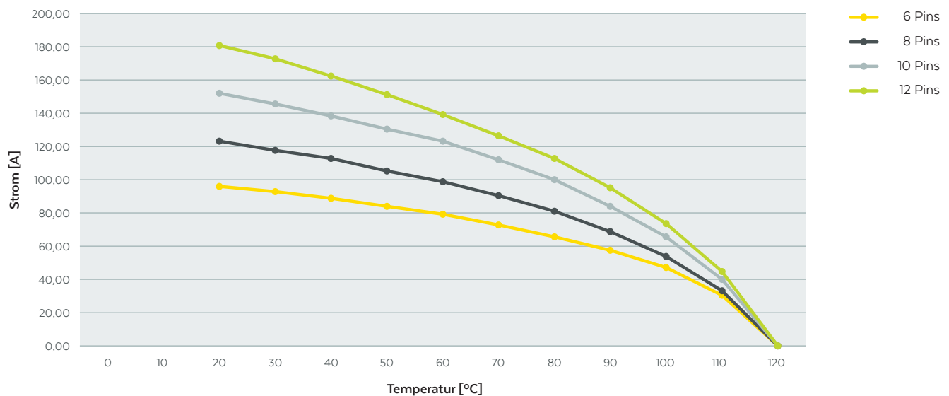
Derating Messung für Power Line massiv zweireihig
