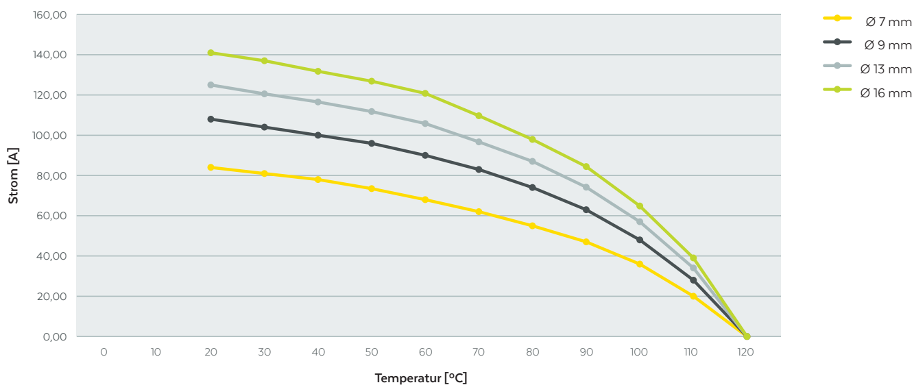
Derating Messung für Power Line SMD
